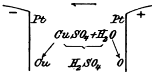
Abb. 59. Elektrolyse von Kupfervitriol-Lösung zwischen Platinelektroden.
